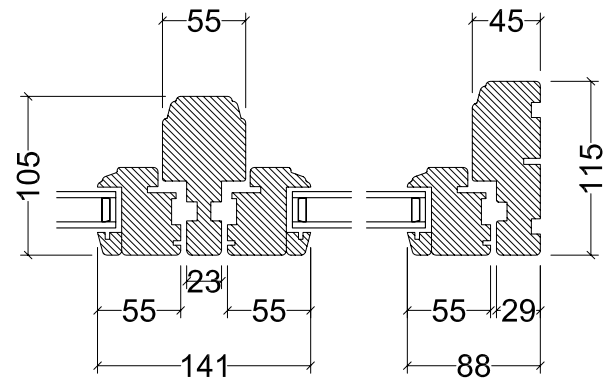
Dannebrog vinduer Lodret snit
