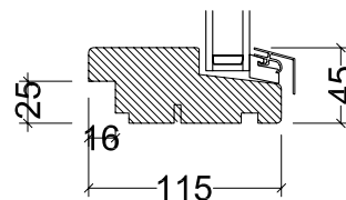
Fals i bundstykke, vindue Lodret snit
