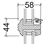
Sprosse Lodret snit
