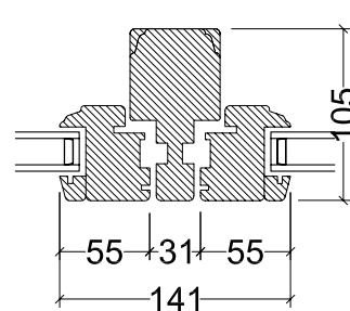
Sprosse Lodret snit
