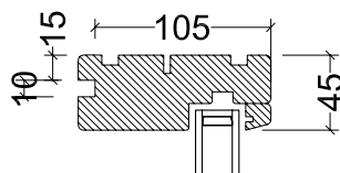
Not i karm Lodret / vandret snit
