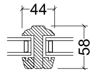
Sprosse Vandret snit
