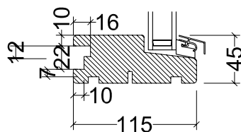
Not i bundstykke, vindue Lodret snit
