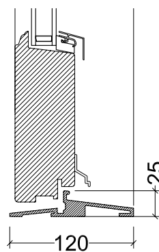
Alubundstykke Indadgående dør Lodret snit
