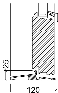
Alubundstykke Udadgående dør Lodret snit
