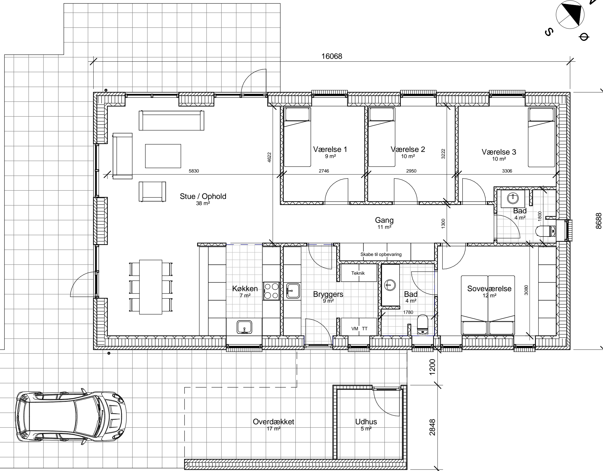
01 Stueplan Mål: 1 : 75
