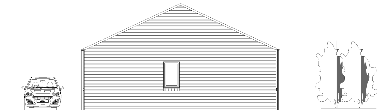
Gavl mod nord 1 : 100
